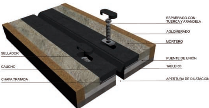
JUNTA PJ-6000 (movimiento 50mm)
