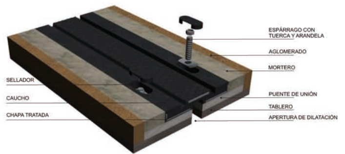
JUNTA PJ-6001 (movimiento 45mm)
