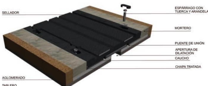
JUNTA PJ-6005 (movimiento 120mm)
